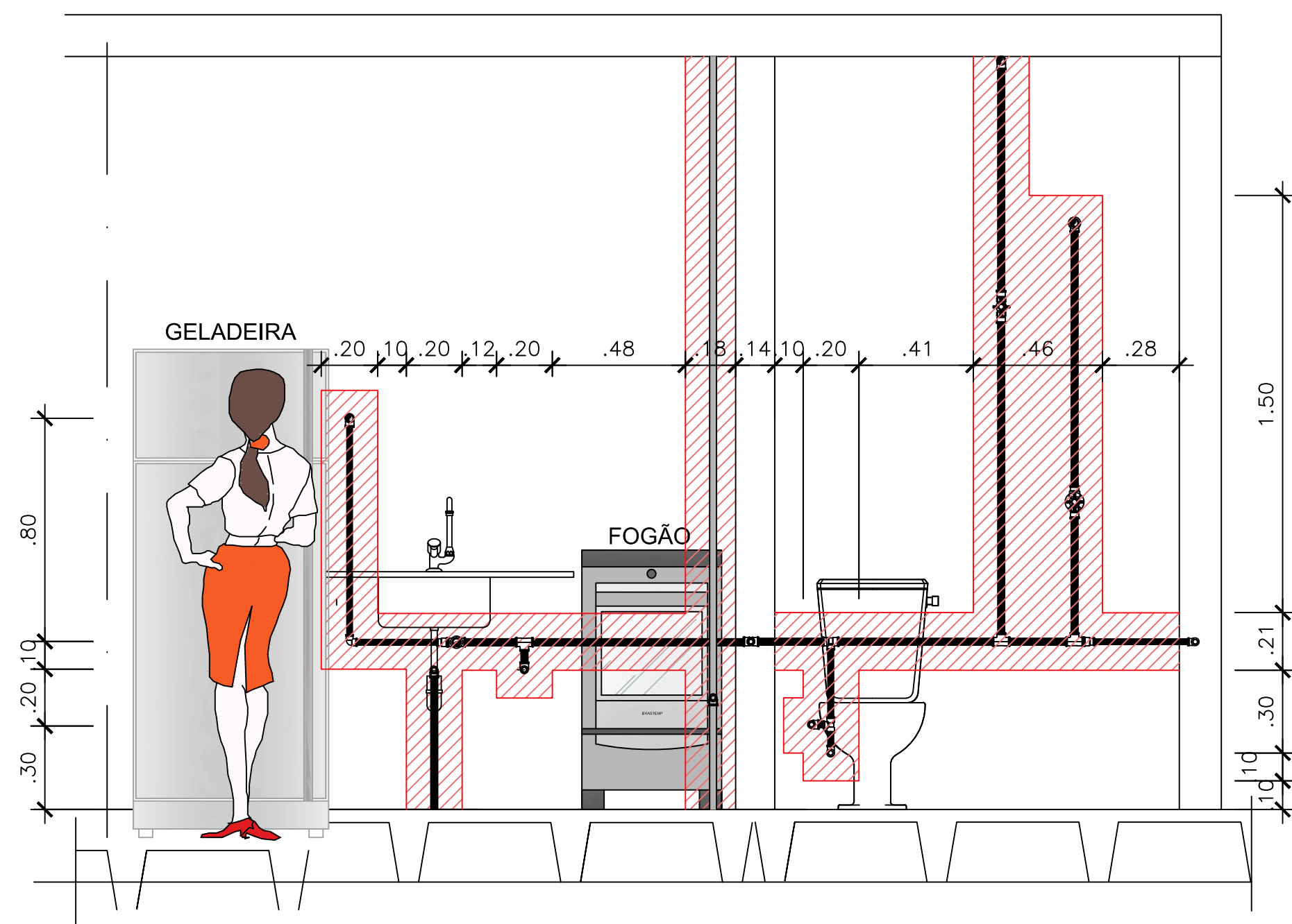
Vista A ESCALA 1/25
